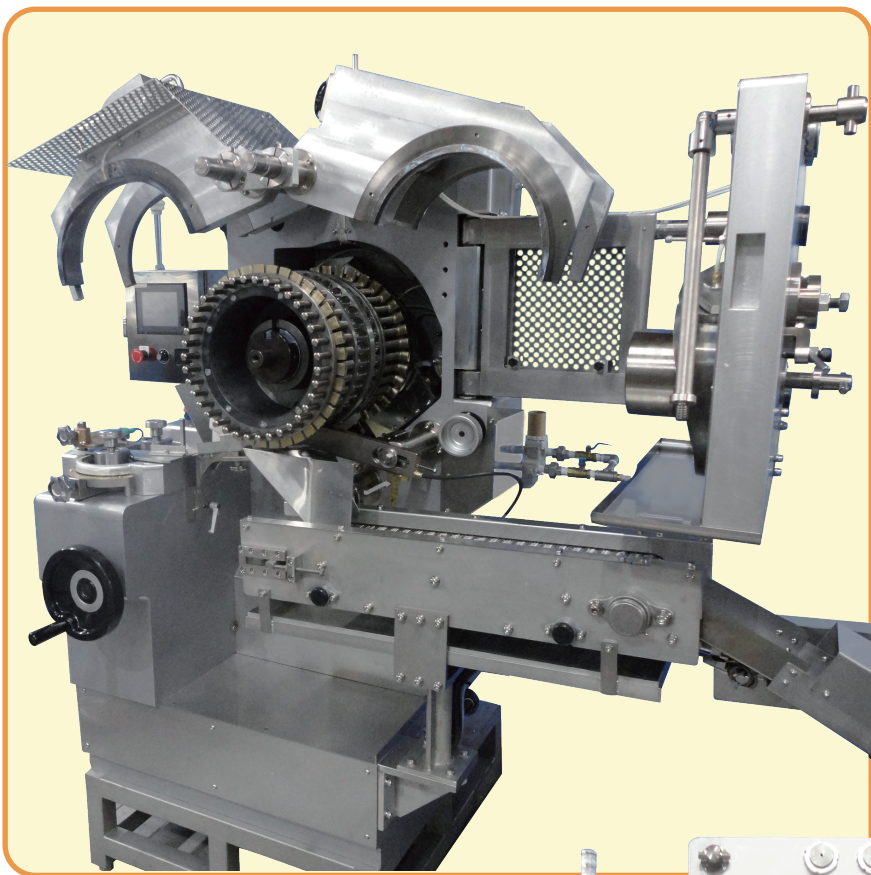
改良型・高速スタンピングマシン (MSP-100II)
